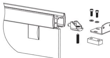
• CKS-SL870-90° Bracket
